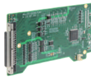
MezIO™-D230/ D220 32/16-CH Isolated Digital I/O
