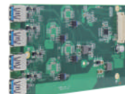
MezIO™-U4-30 4 x USB 3.1 Gen 1 Ports
